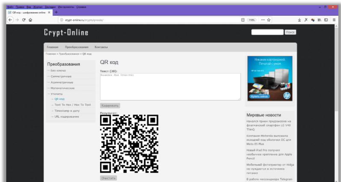
Рисунок 1.1. Создание QR-кодов.
